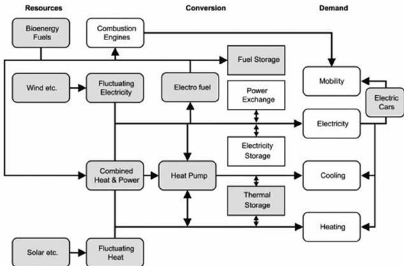
Holistische benadering van energienetwerken (Connolly et al 2016)
